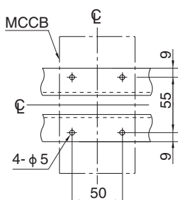
安装开孔尺寸 (角铁安装时)
