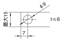
端子部详图
