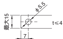
连接导体加工图
