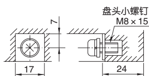
端子部详图
