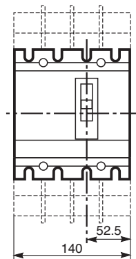
4极产品
