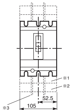
3极产品
