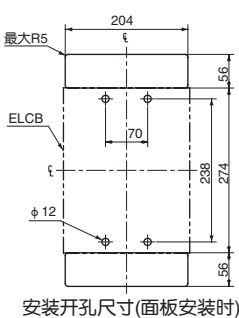
安装开孔尺寸(面板安装时)
