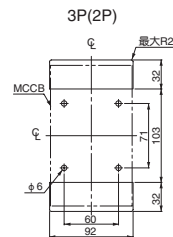
安装开孔尺寸(面板安装时)
