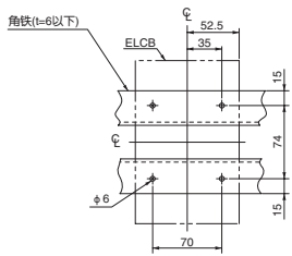
安装开孔尺寸(角铁安装时)
