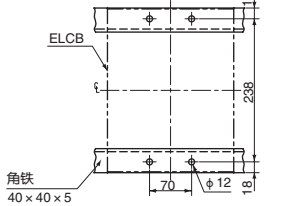
安装开孔尺寸(角铁安装时)
