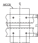
安装开孔尺寸(角铁安装时)
