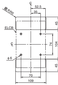
安装开孔尺寸(面板安装时)
