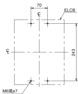
安装开孔尺寸
