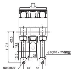
【从电源侧看】
