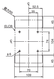
安装开孔尺寸(面板安装时)
