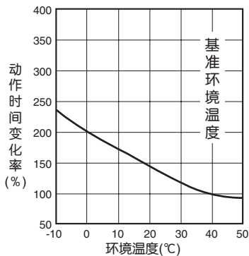
●温度补偿曲线
