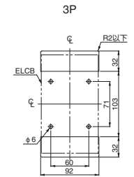
安装开孔尺寸(面板安装时)
