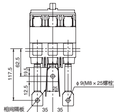
【从电源侧看】
