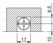
端子部详图
