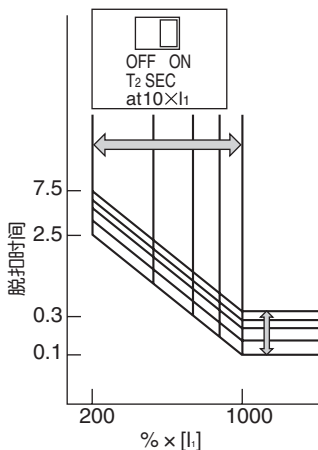
电流设定范围, 额定电流 I_t 的200%~1000%。
