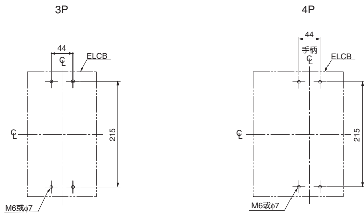
安装开孔尺寸
