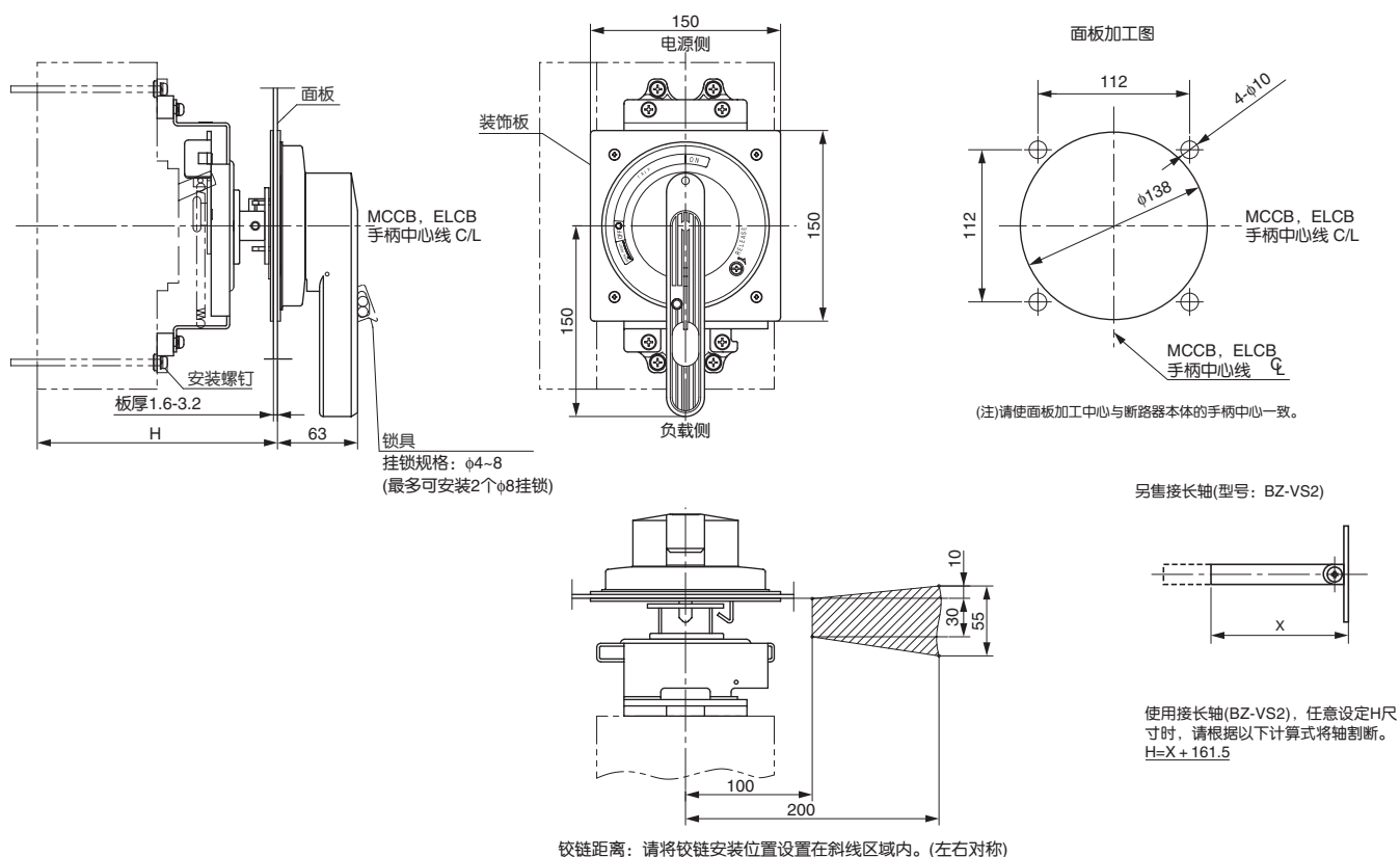
(c)-3 外形及安装方法(BW9V0HA, BW9V0JA)
