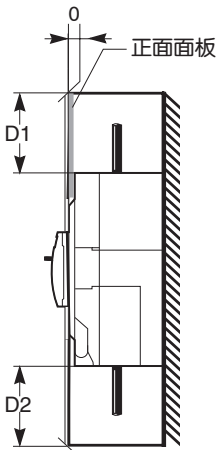
MCCB与正面面板之间的最小距离
