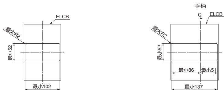
面板开孔尺寸
