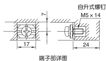
端子部详图
