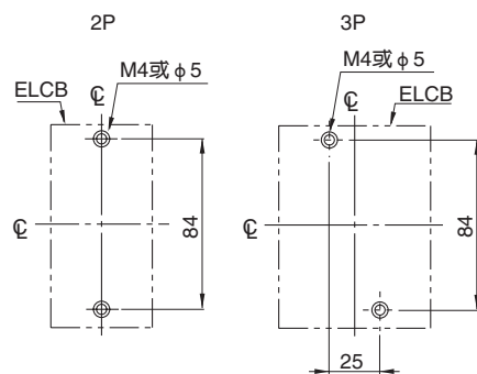
安装孔尺寸
