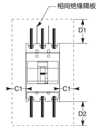
MCCB与脱扣、顶部或底部或侧面面板之间的最小距离
