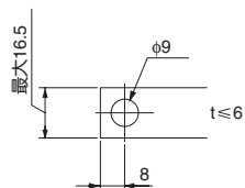
连接导体加工图
