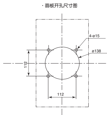
· 面板开孔尺寸图
