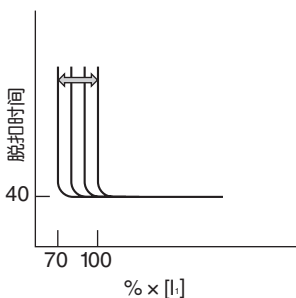
预报警电流设定范围, 额定电流 I_t 的70%~100%。 预脱扣报警动作时间, 40s恒定。
