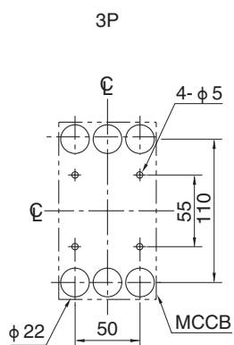
安装开孔尺寸 (面板安装时)
