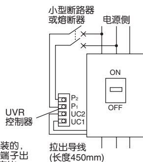
UVR控制器的另行安装
