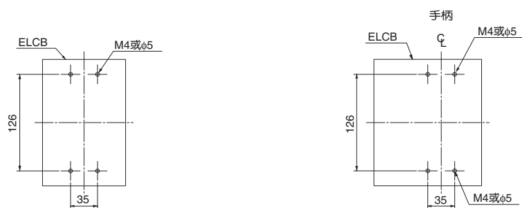
安装开孔尺寸
