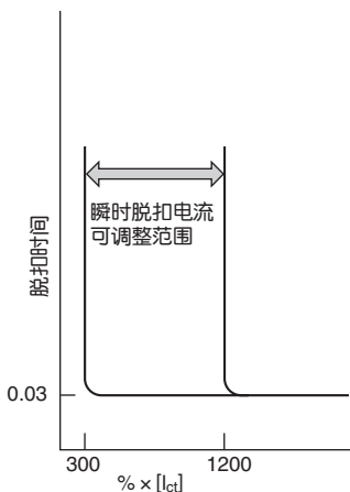
电流设定范围, 额定一次电流 I_{ct} 的300%~1200%。
