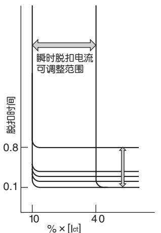
电流设定范围, 额定一次电流的10%~40%。
