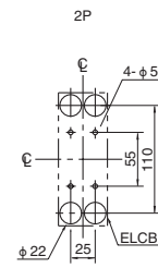
安装开孔尺寸 (面板安装时)
