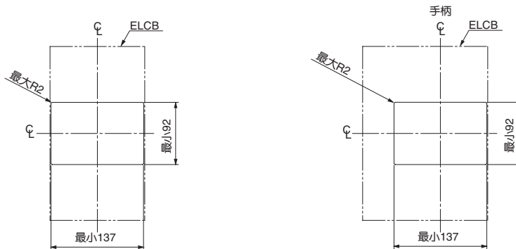
面板开孔尺寸
