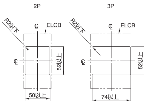
面板钻孔尺寸
