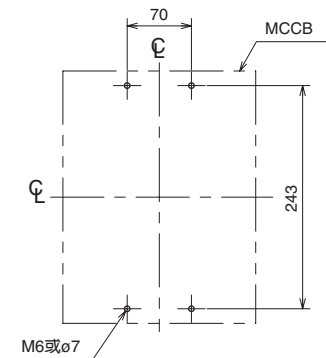
安装开孔尺寸
