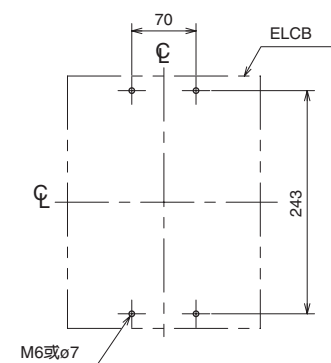
安装开孔尺寸
