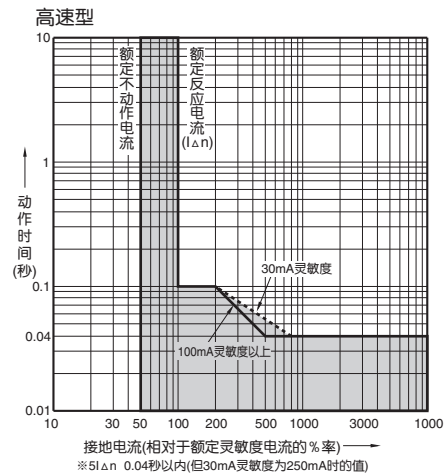
●漏电脱扣特性
