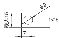
连接导体加工图
