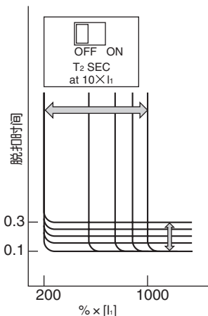
电流设定范围, 额定电流 I_t 的200%~1000%。
