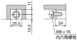
端子部详图
