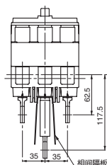
【从负载侧看】
