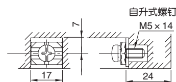
端子部详图
