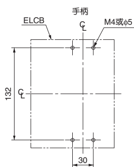
安装开孔尺寸
