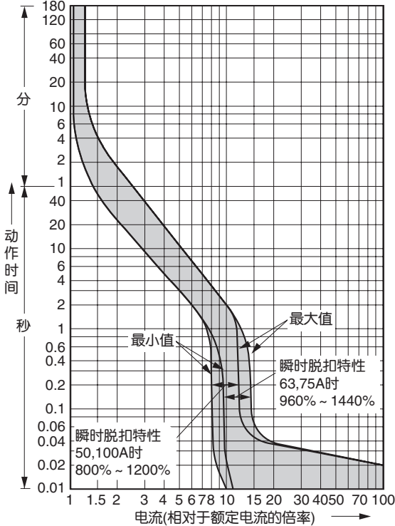
●动作特性曲线 一般配线用瞬时固定型
