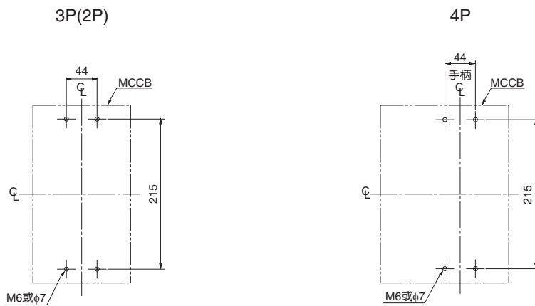
安装开孔尺寸
