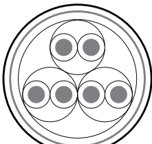
3对电缆的结构图例
