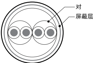
2对电缆的结构图例
