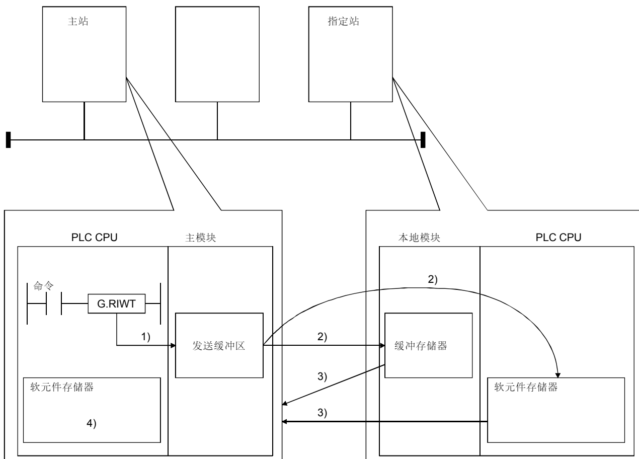
(a) RIWT 指令的操作图
