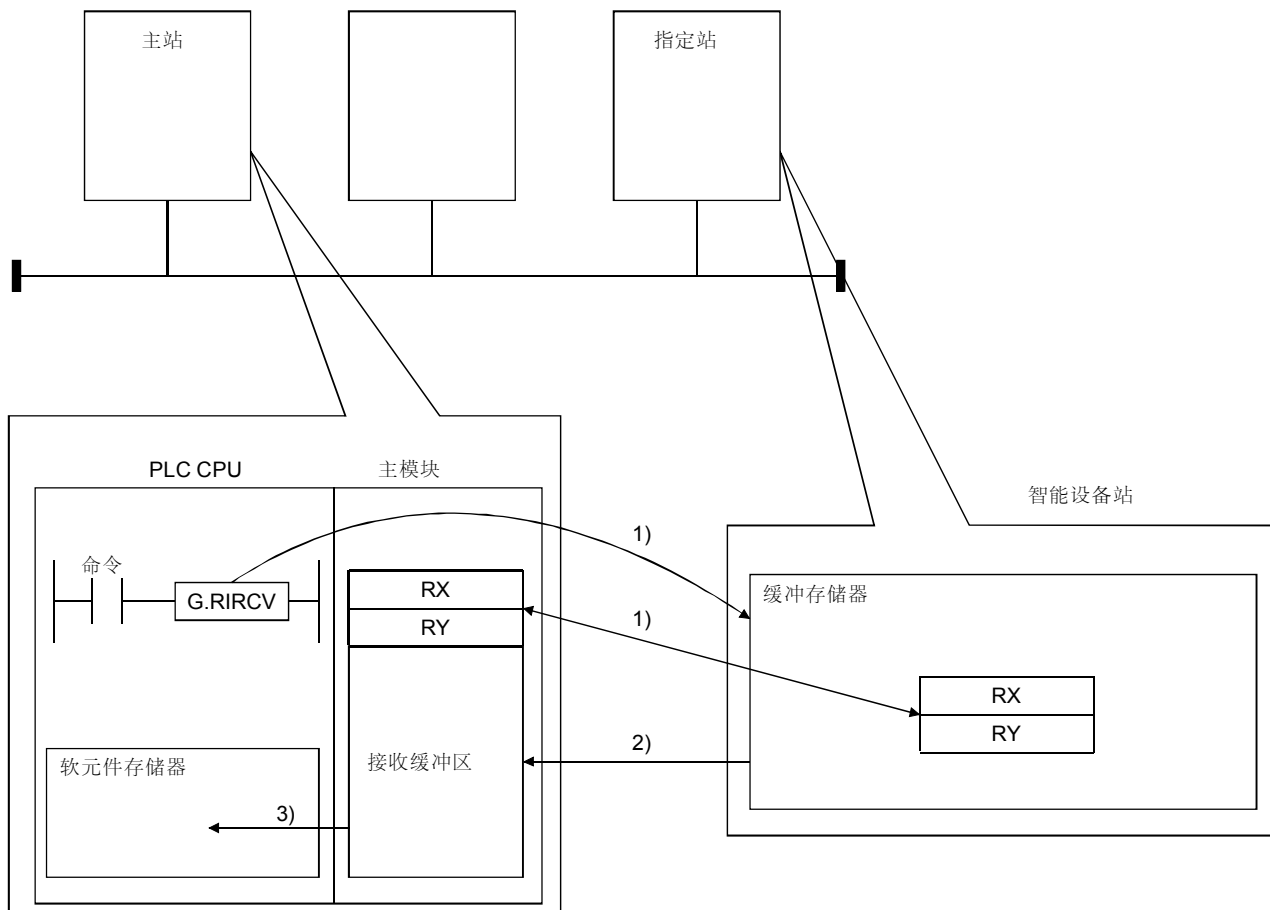
(a) RIRCV 指令的运行图
