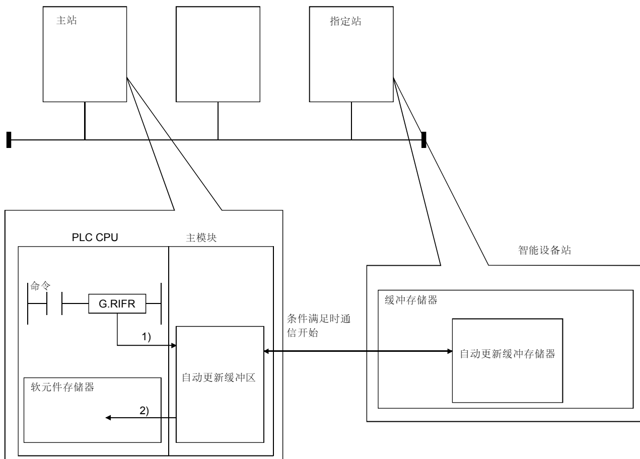
(a) RIFR 指令的运行图
