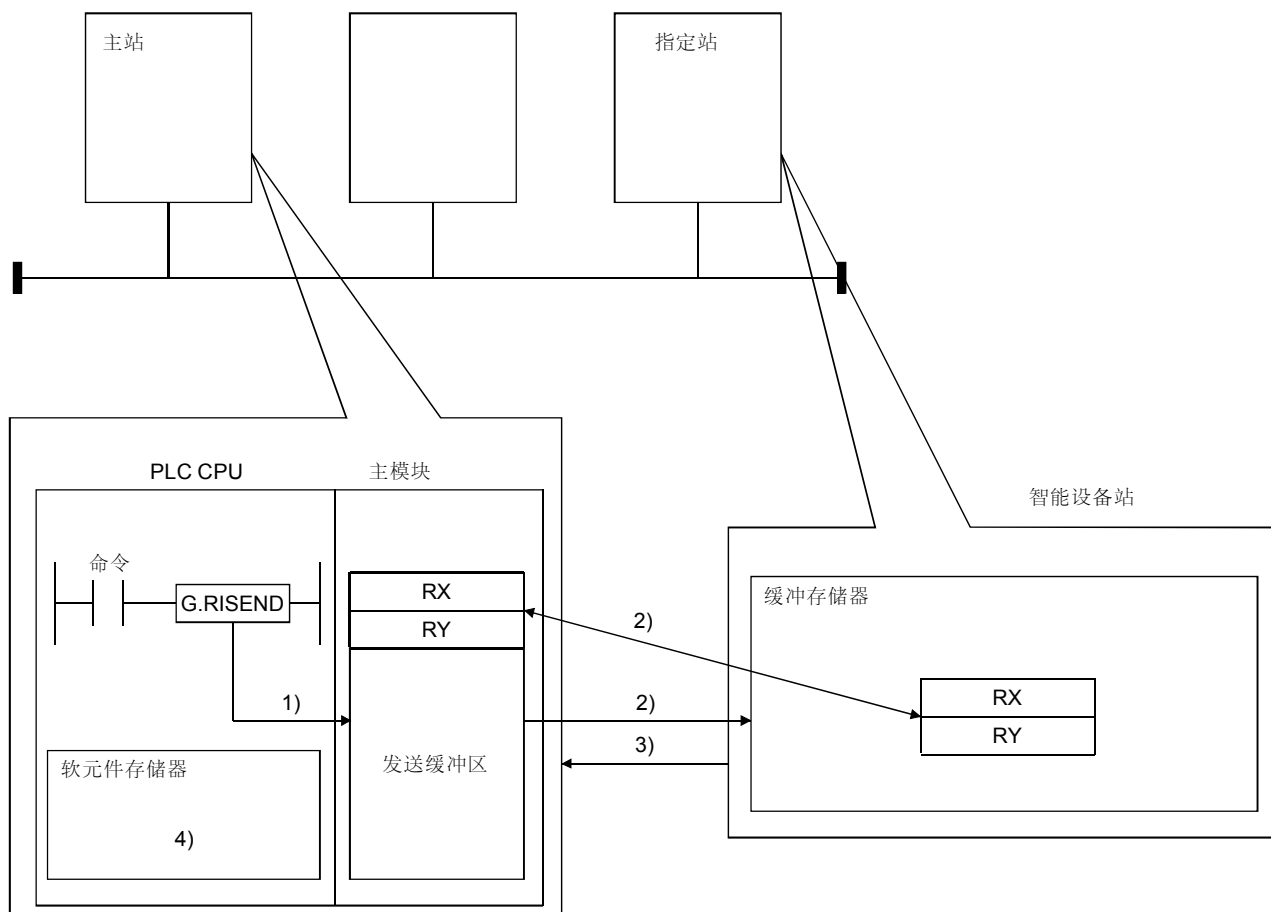
(a) RISEND 指令的运行图
