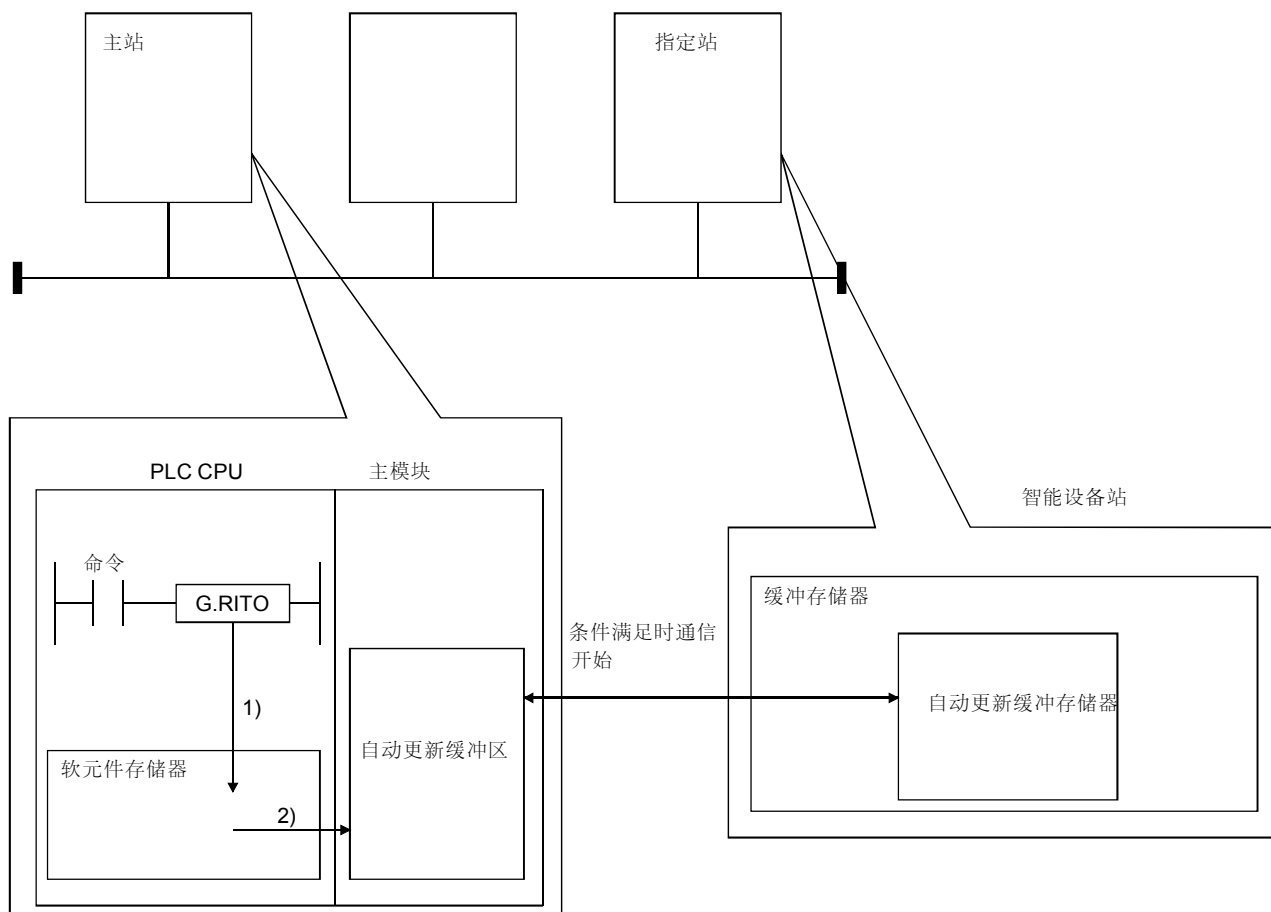
(a) RITO 指令操作图
