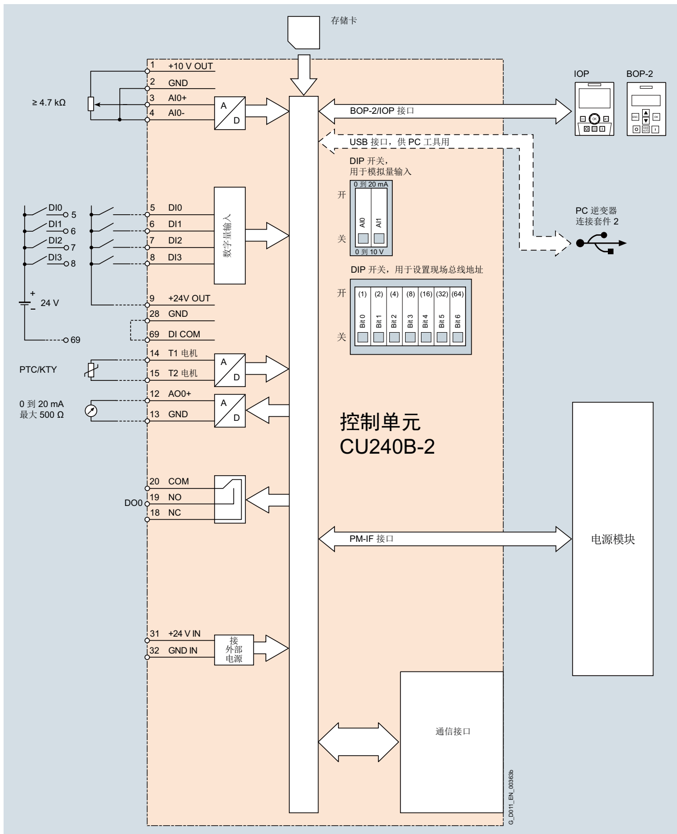
CU240B-2 系列控制单元的接线图
