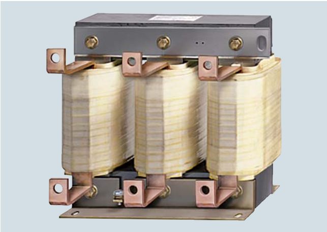
输出电抗器，适用于功率模块 PM240 FSGX
